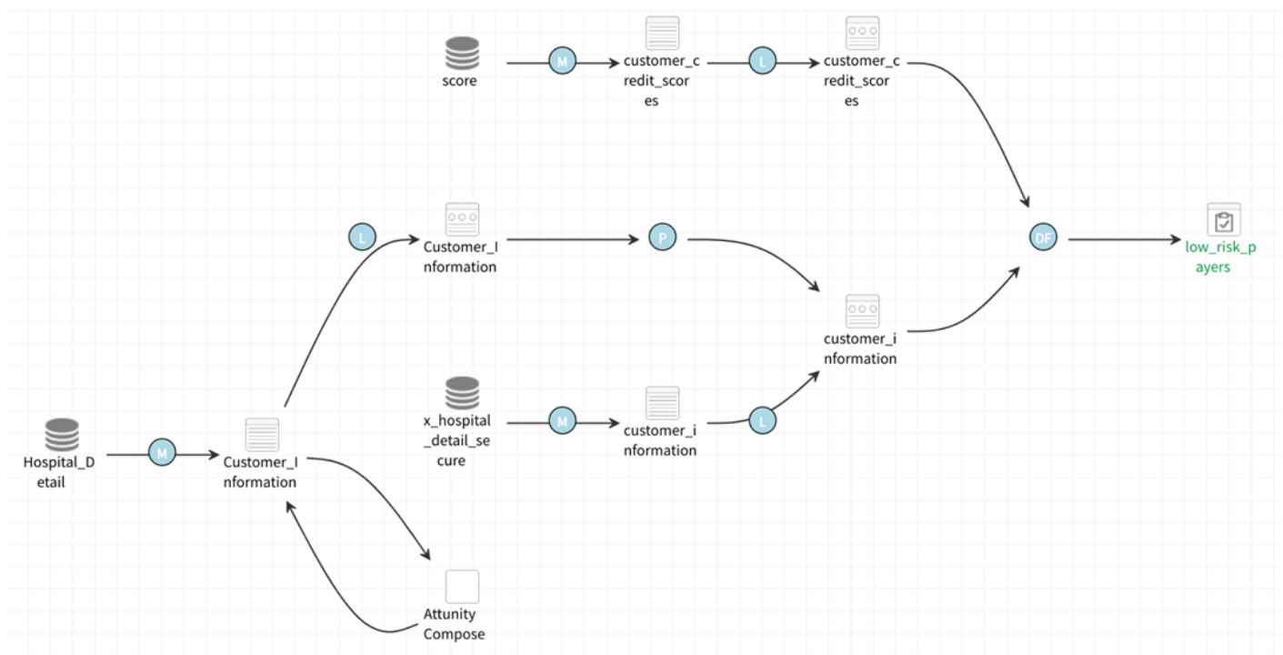
Figura 1: Exemplo de visualização de um grafo de exibição de linhagem de dados.
