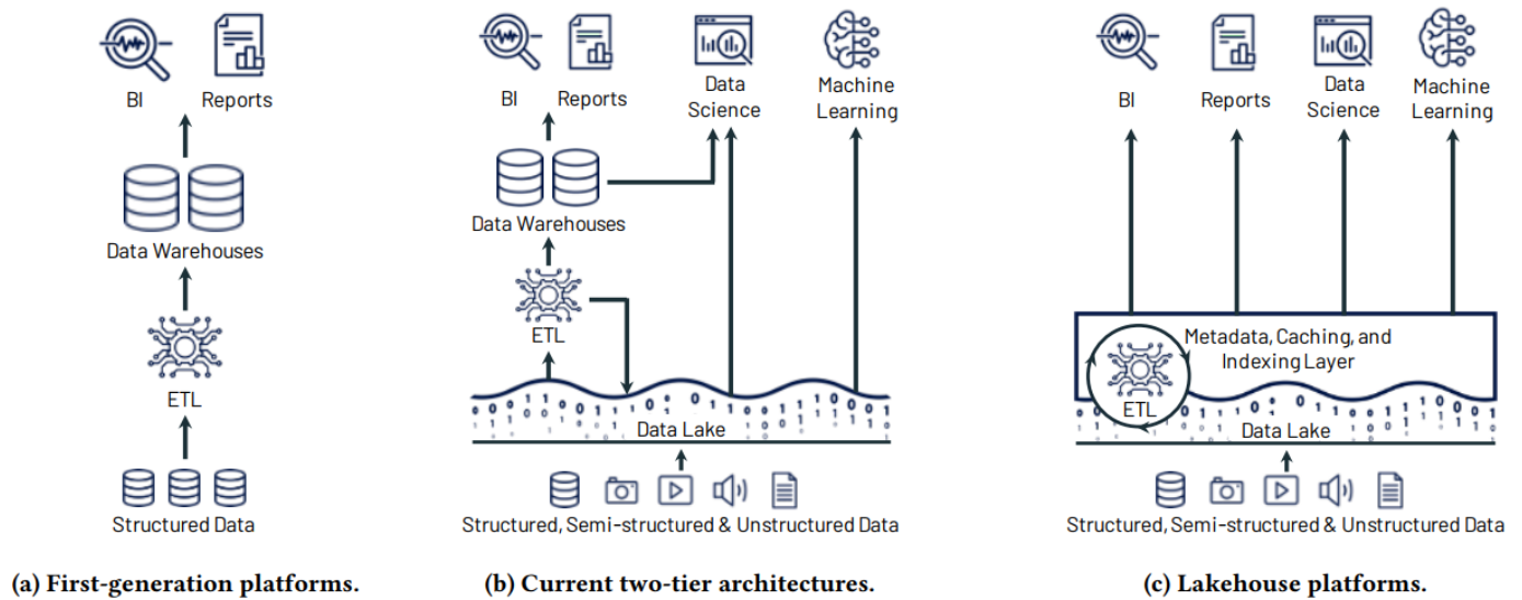
Figura 1: Evolução das arquiteturas de plataforma de dados. Fonte: (ARMBRUST, GHODSI, XIN e ZAHARIA, 2021).
